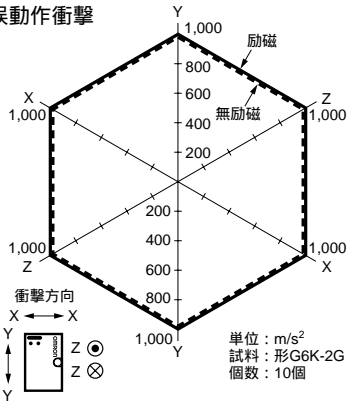
誤動作衝撃
