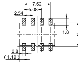
プリント基板加工寸法 (TOP VIEW) 寸法公差は±0.1mmです。
