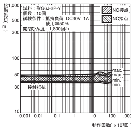
電気的耐久性 (接触抵抗) *1
