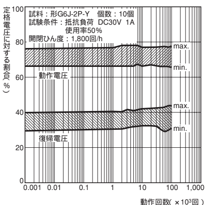
電気的耐久性 (動作・復帰電圧) *1
