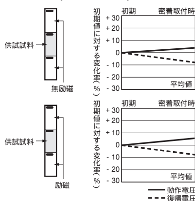
磁気干渉 (リレー相互)
