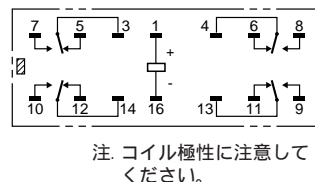
端子配置/内部接続図 (BOTTOM VIEW)
