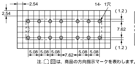
プリント基板加工寸法 (BOTTOM VIEW) 寸法公差は±0.1mmです。
